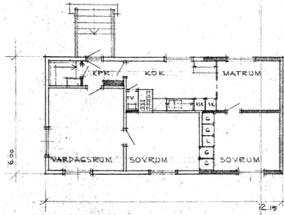
BOTTENVÅNING
