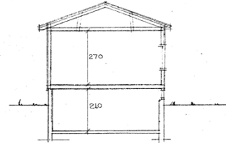
SEKTION
