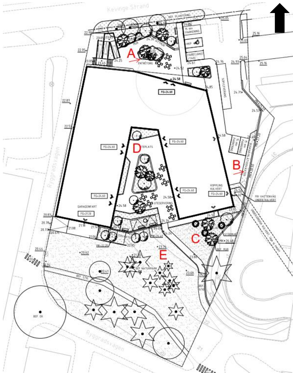
Figur 8. Placering av planerade och föreslagna LOD-åtgärder.
