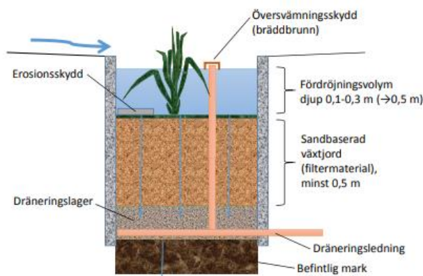
Figur 6. Principskiss av nedsänkt växtbädd. Illustration av WRS. 16
