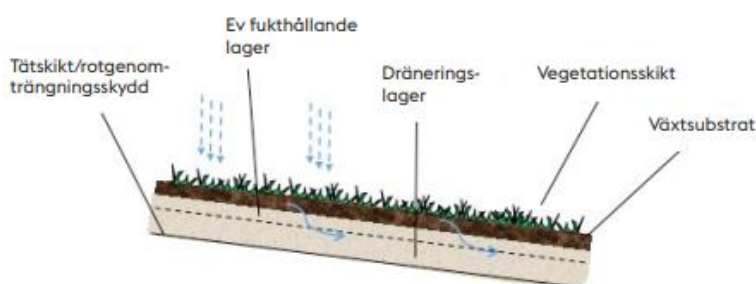
Figur 7. Principskiss av vegetationsbeklätt tak. Dräneringslagret vilar direkt på tätskiktet på för takkonstruktionen. Ifall taket skulle bli övermättat så rinner överskottsvattnet via dräneringslagret till hängrännor och stuprör. Illustration av WRS.
