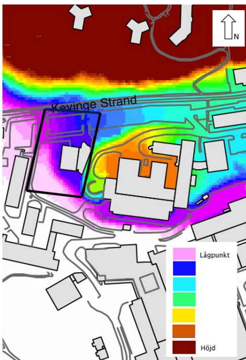
Figur 9. Höjdkarta över utredningsområdet. Kartan mottagen från Danderyds kommun.
