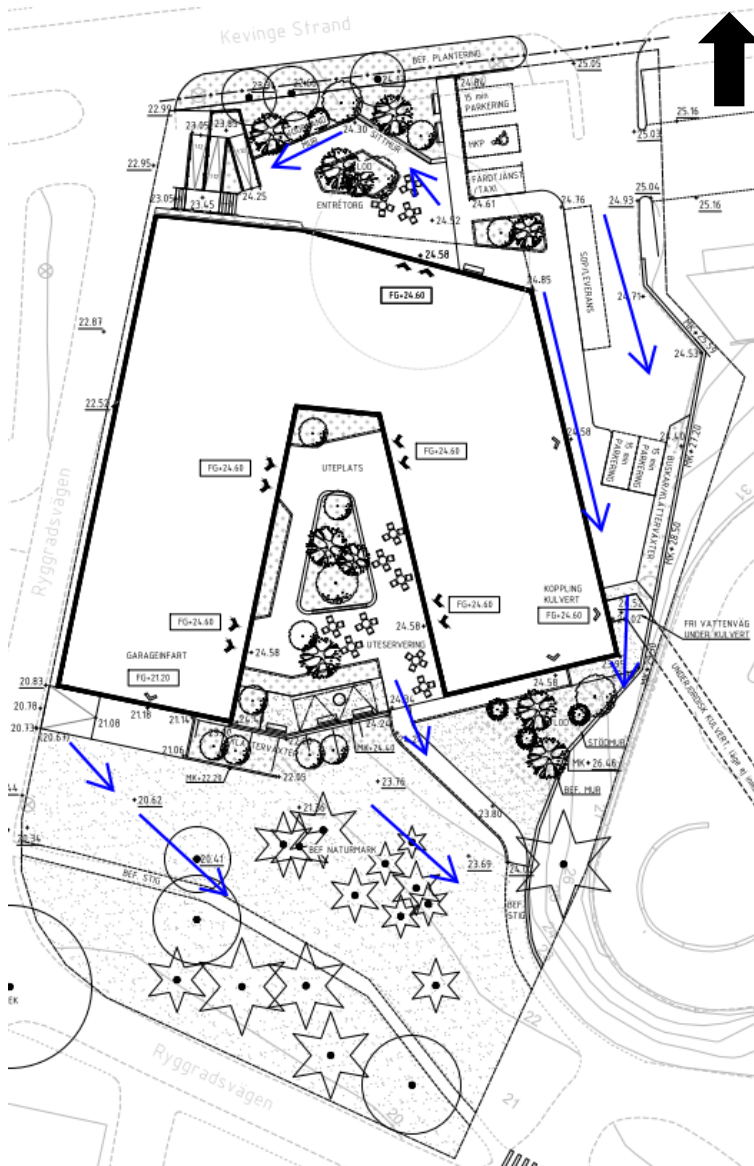
Figur 12. Principskiss av ytliga avrinningsvägar efter omdaning. Den röda markeringen visar en mur där släpp till planteringsytan bör finnas.
