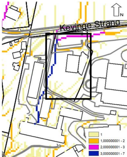
Figur 10. Skyfallskarta för ytavrinningen. Den svarta rutan markerar utredningsområdet. Kartan mottagen från Danderyds kommun.
