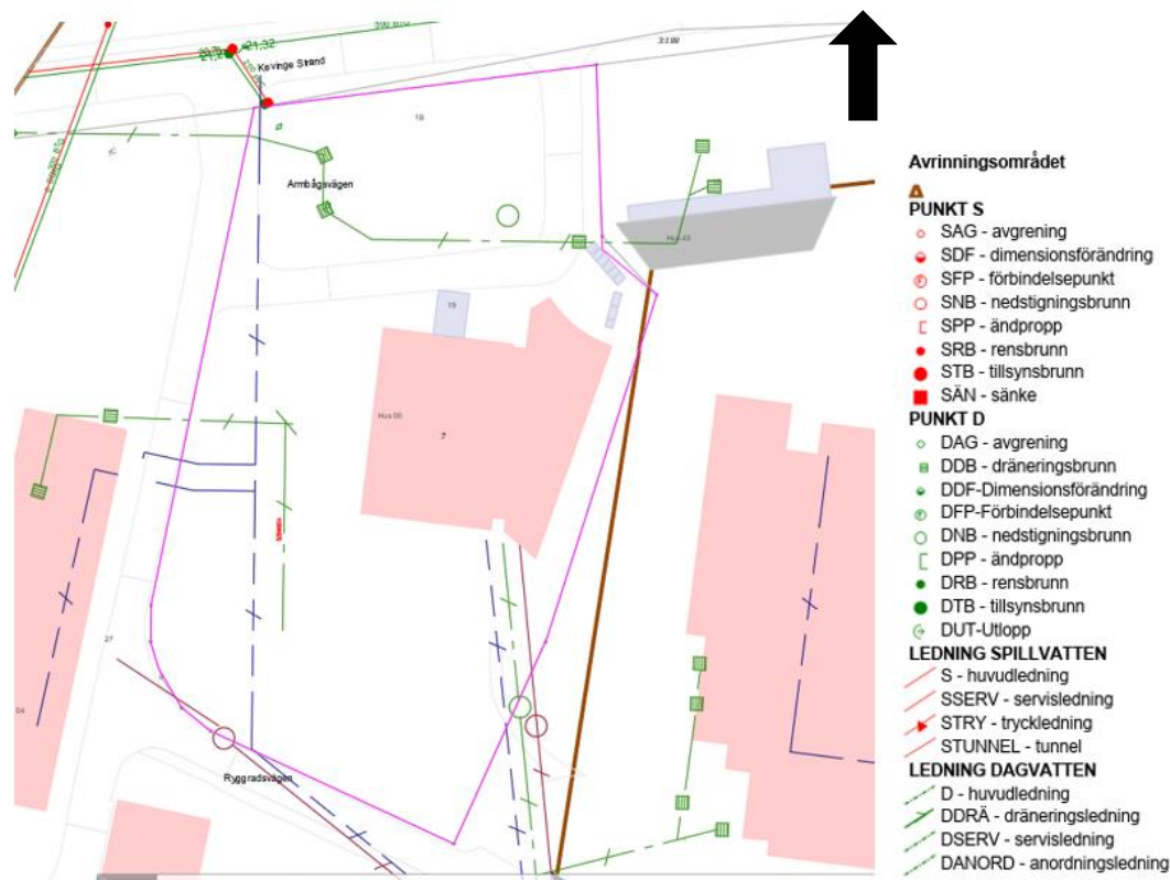
Figur 5. Sammanslagning av Danderyds kommun ledningskarta och ledningskarta från WRS 12 . Den lila linjen avser utredningsområdet.
