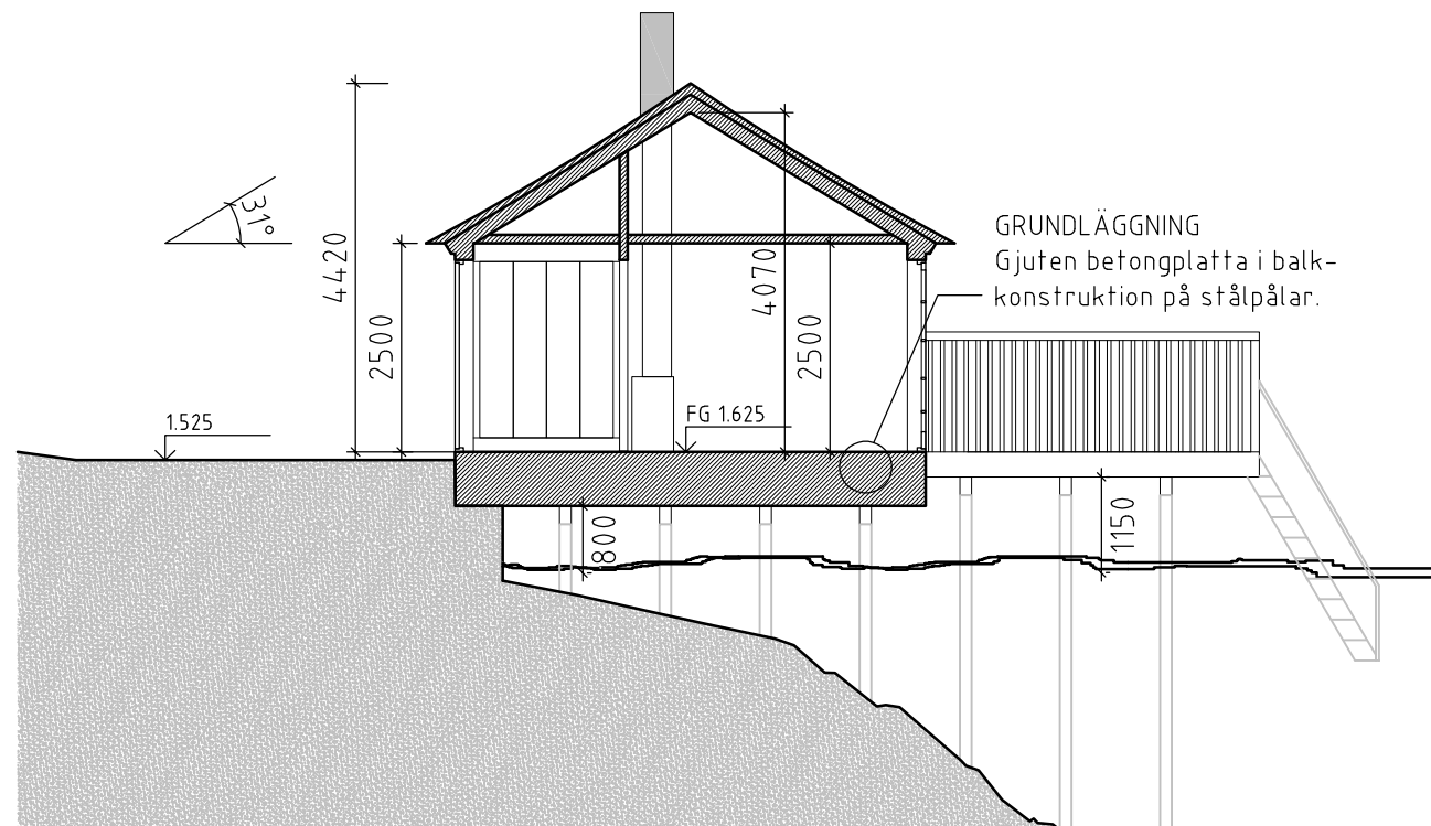
SEKTION AA
