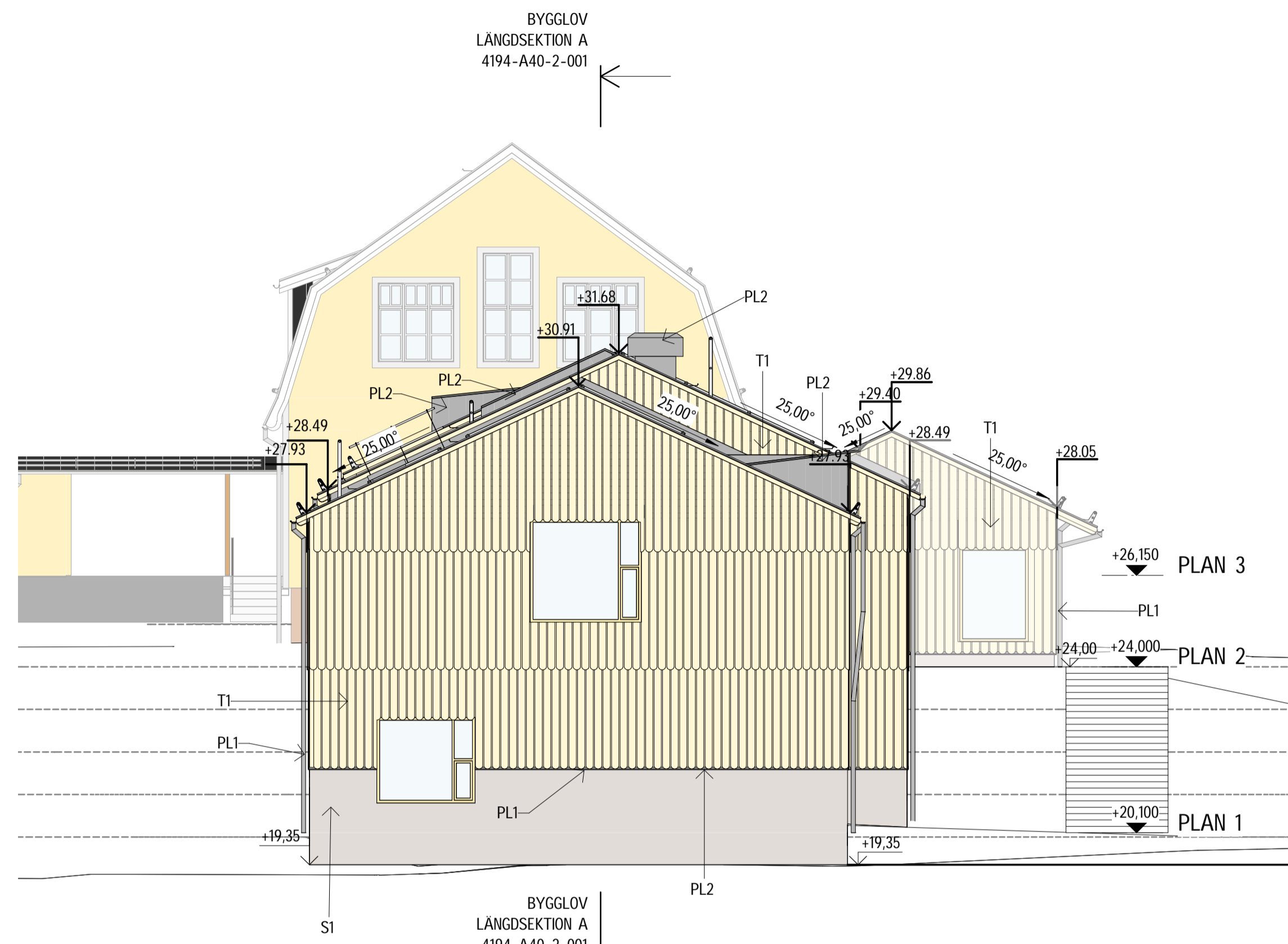
FASAD MOT NORR
