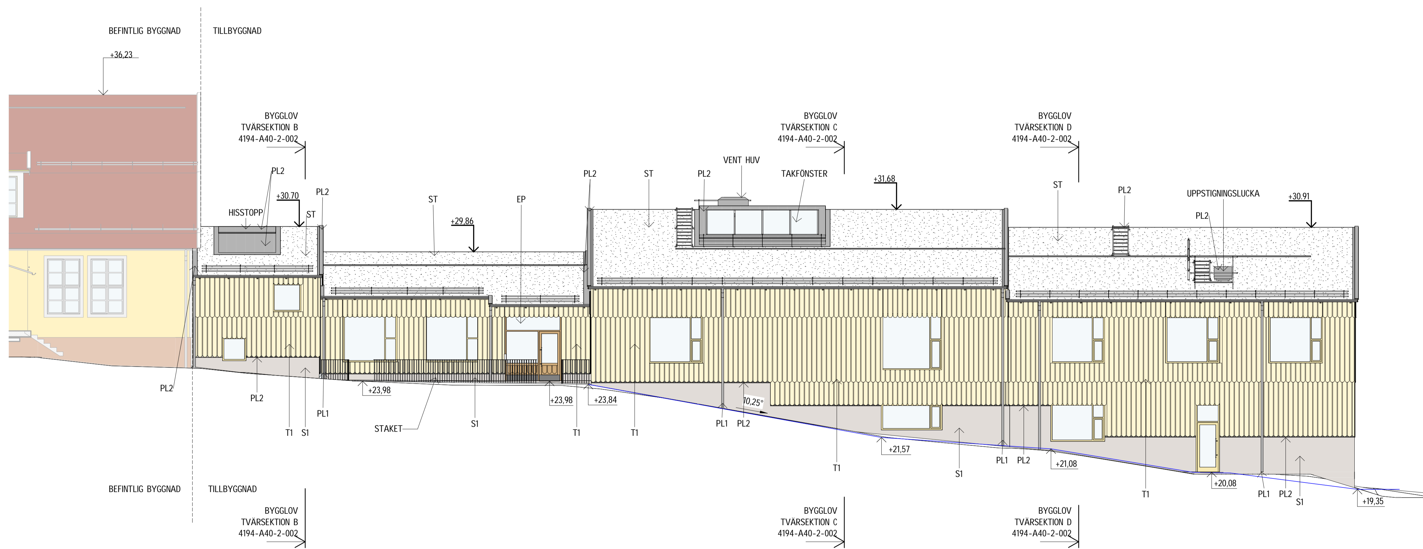
FASAD MOT ÖST
