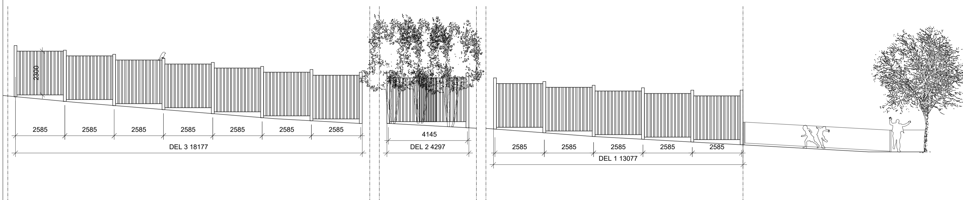
BULLERSKYDDSPLANK ELEVATIONER SKALA 1:100/A1
