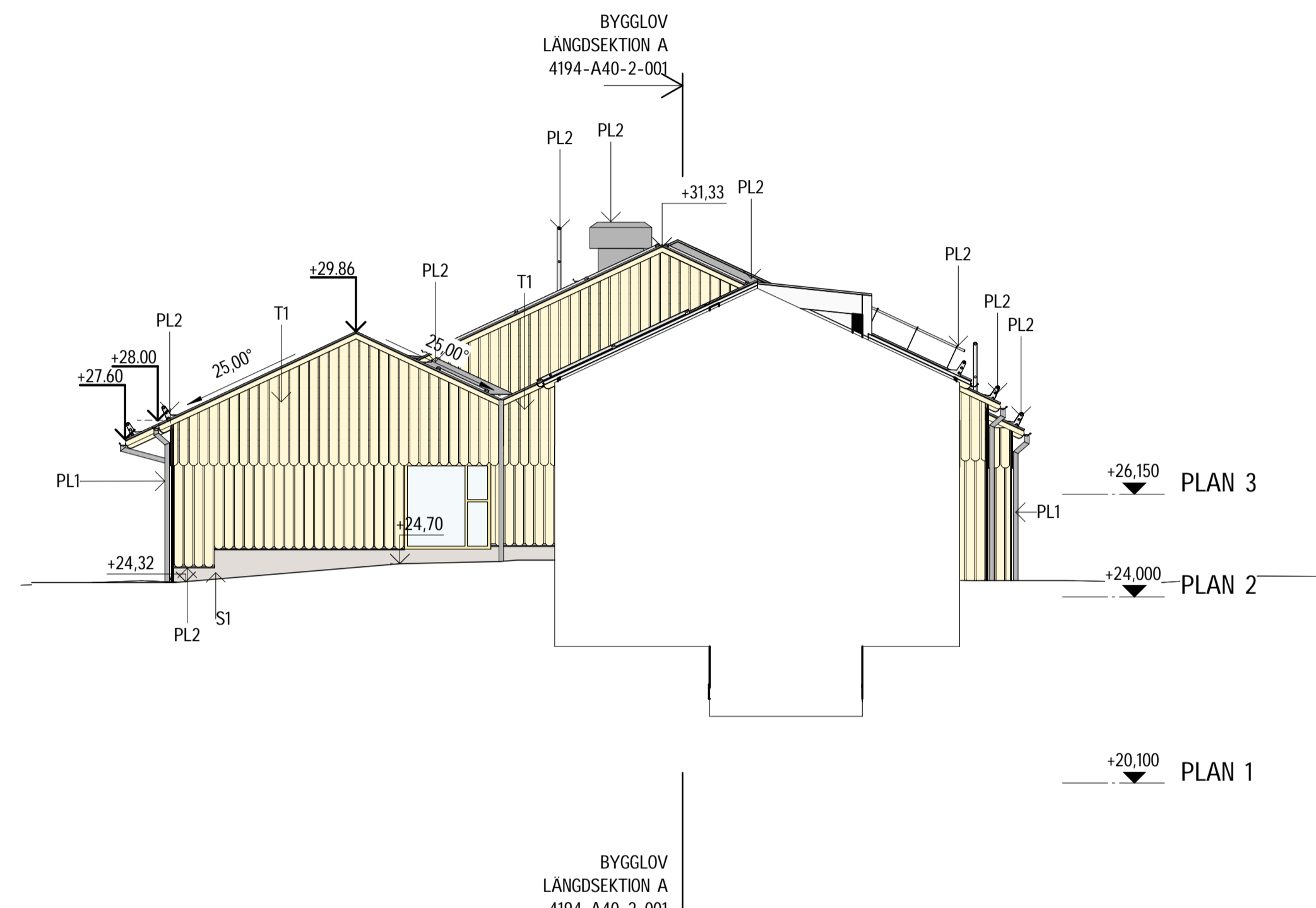
FASAD MOT SYD
