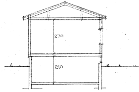
SEKTION
