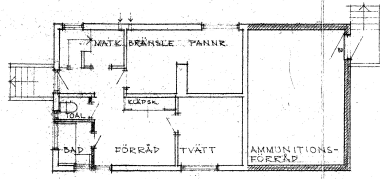
KÄLLARPLAN
