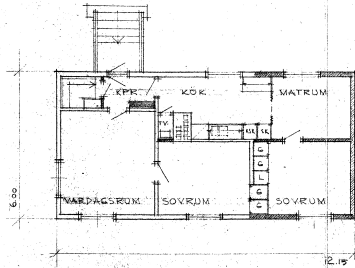
BOTTENVÄNING
