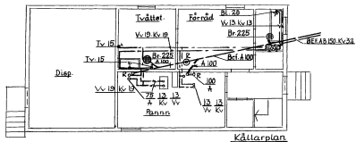
Källarplan
