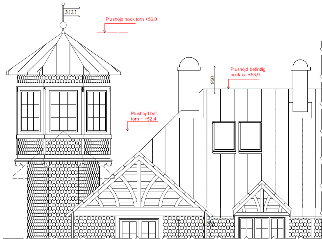
Fasad mot norr Skala 1:50
