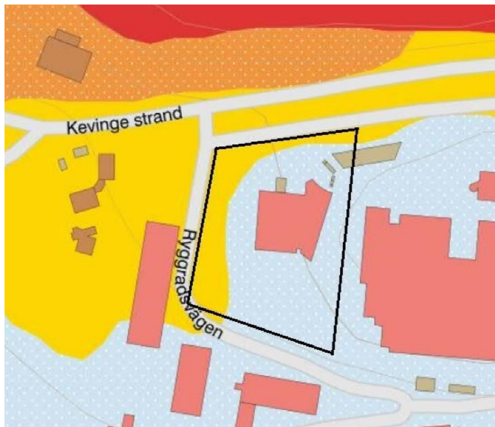
Utsnitt ur SGU:s jordartskarta från PM Geoteknik Sjukhuset 7, Tyréns 2020-10-13, med ungefärligt utredningsområde markerat. Ljusblå prickig yta visar sandig morän och gul färg visar glacial lera.
