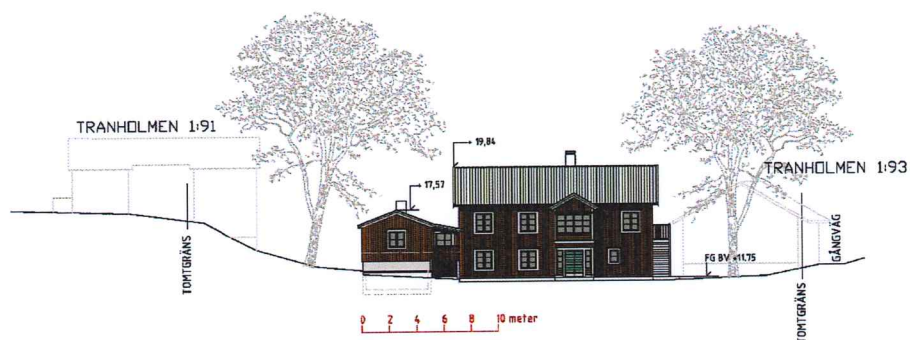
Sektion BB, väster till vänster i bild, öster till höger (se markering på situationsplan).
